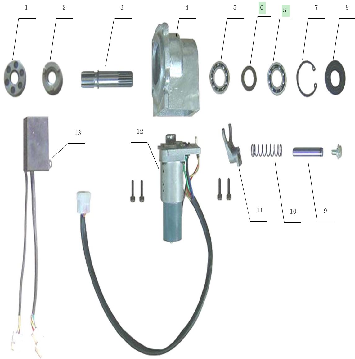
11、二四转换总成 2WD-4WD
