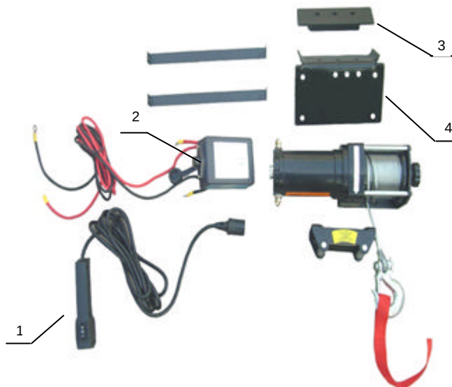
VI 36,WINCH ASSY
