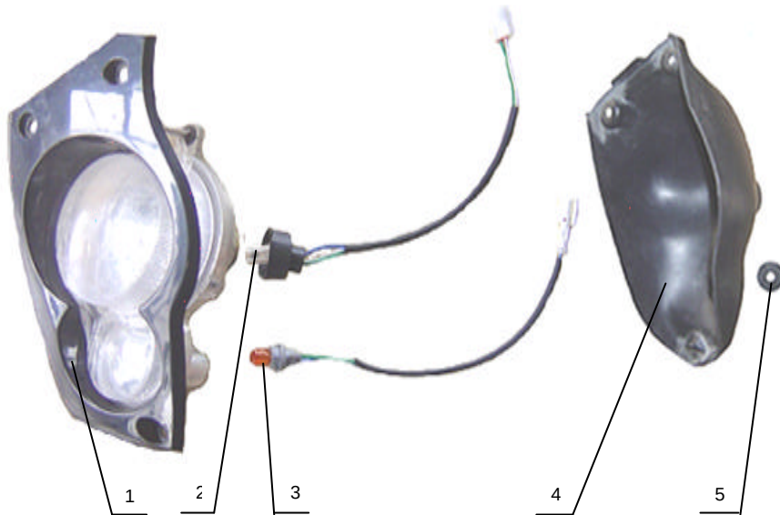
VI 26 ,HEAD LIGHT
