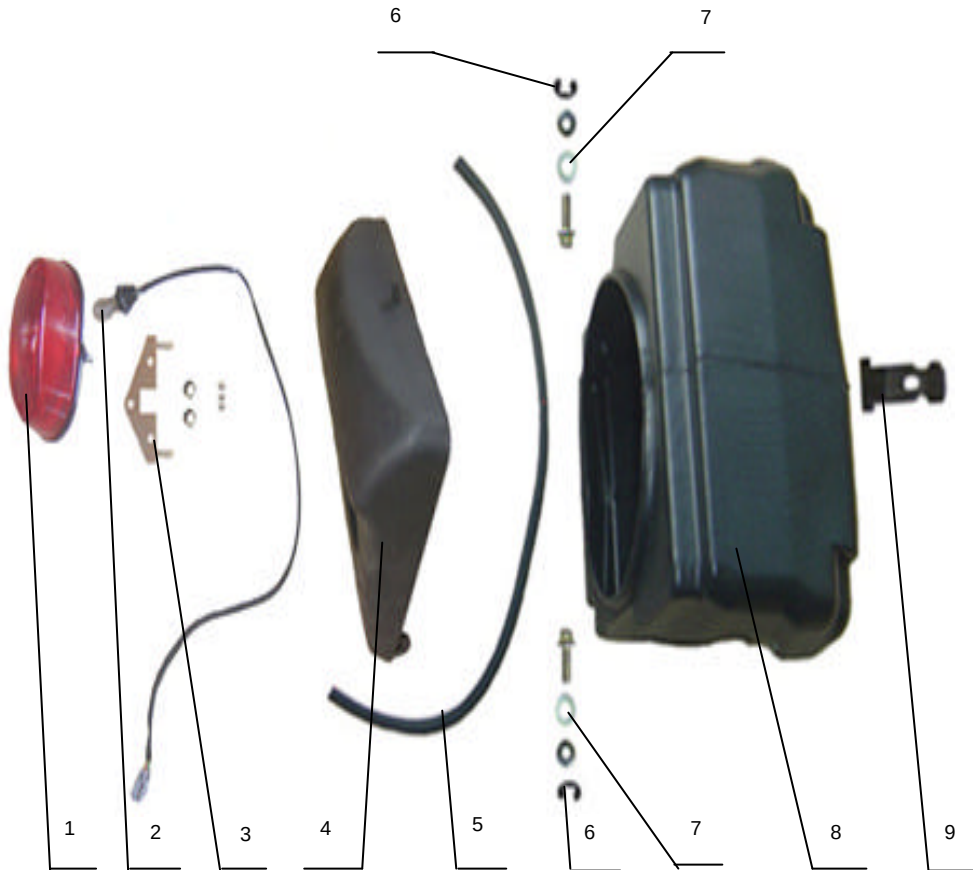
VI 23 ,KIT BOX ASSY
