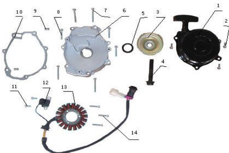
E5 ? ? ? ? ? Alternator
